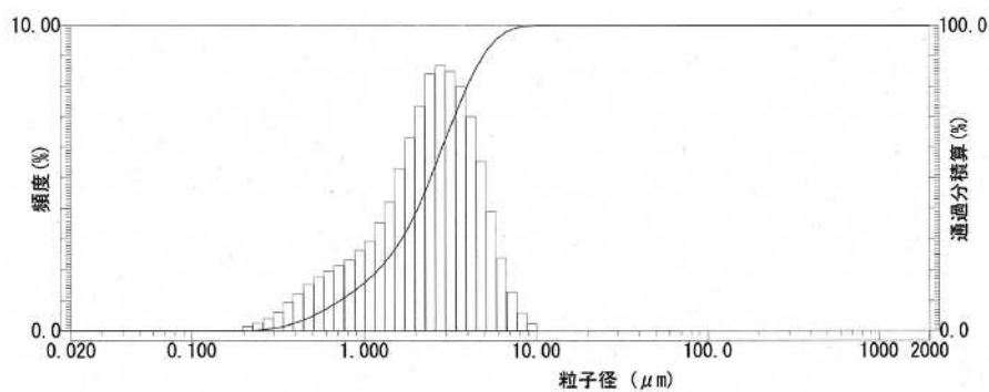
粒度分布
